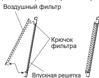
Впускная решетка
